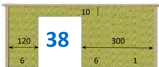
Baie vitrée h 210* 180 cm désaxée - réversible
