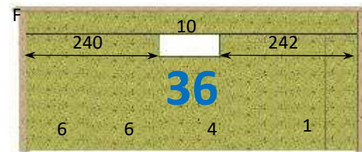
Imposte centrée h 40 x 118 cm
